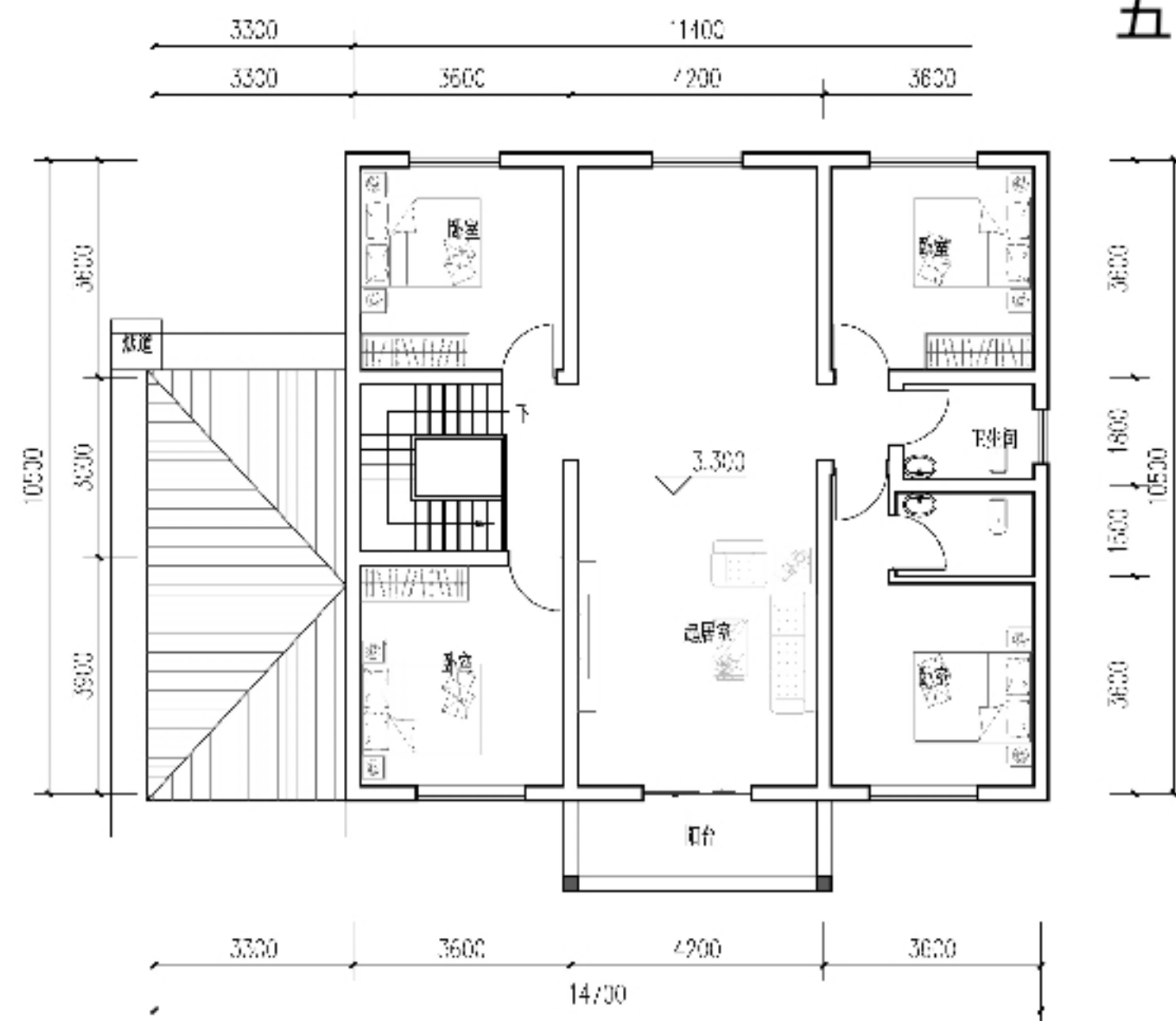
二層平面圖 1:100
