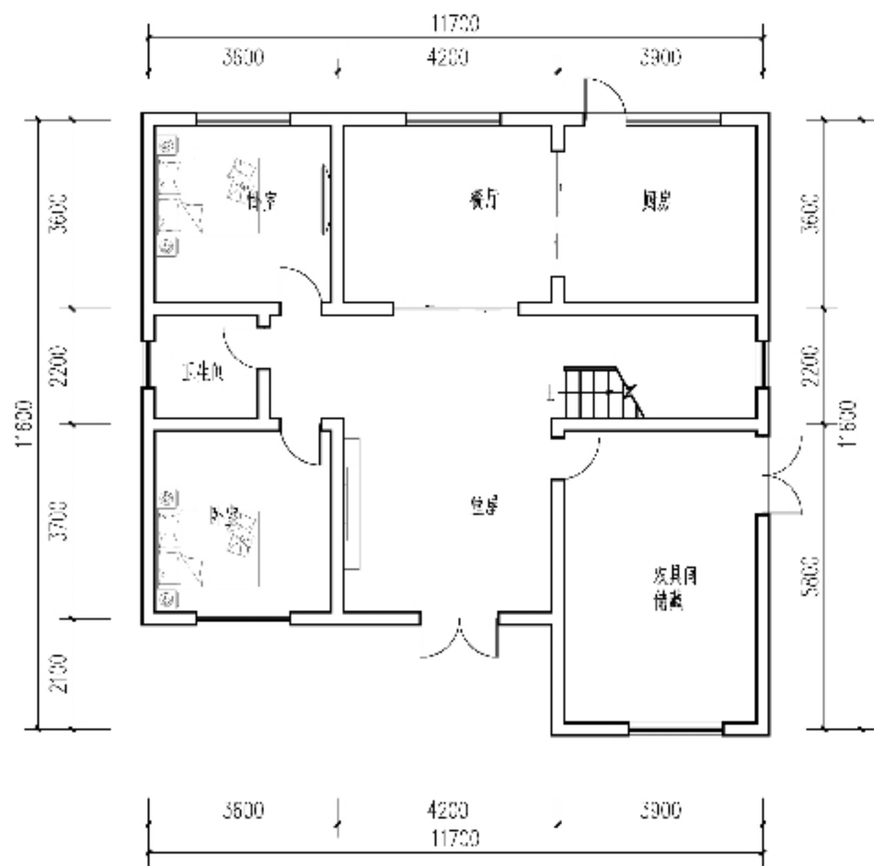
一层平面图 1:100 本层建筑面积: 124.99m 2
