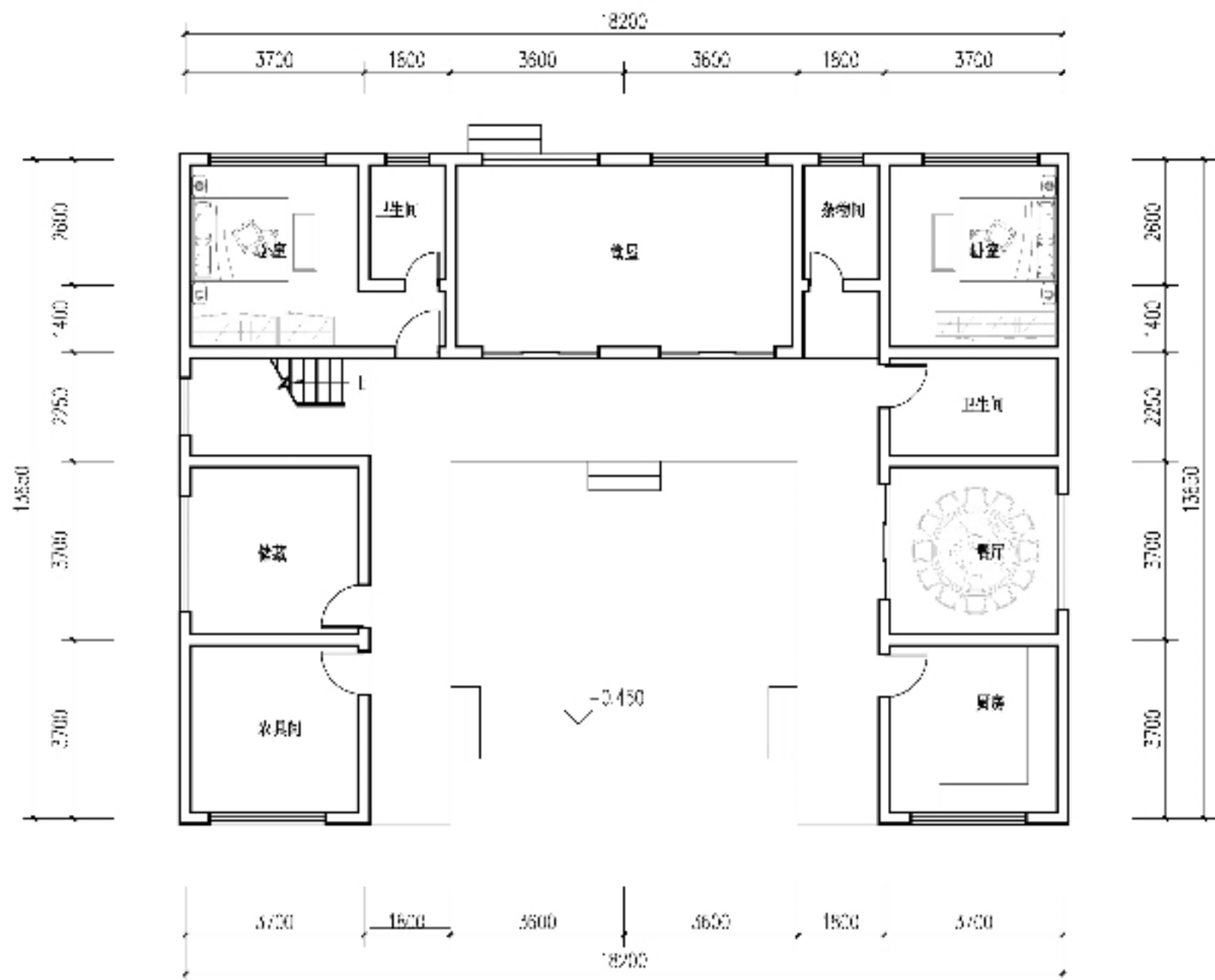
一层平面图 1:100
