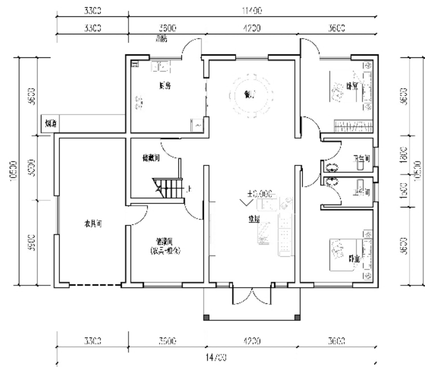
一层平面图 1:100
