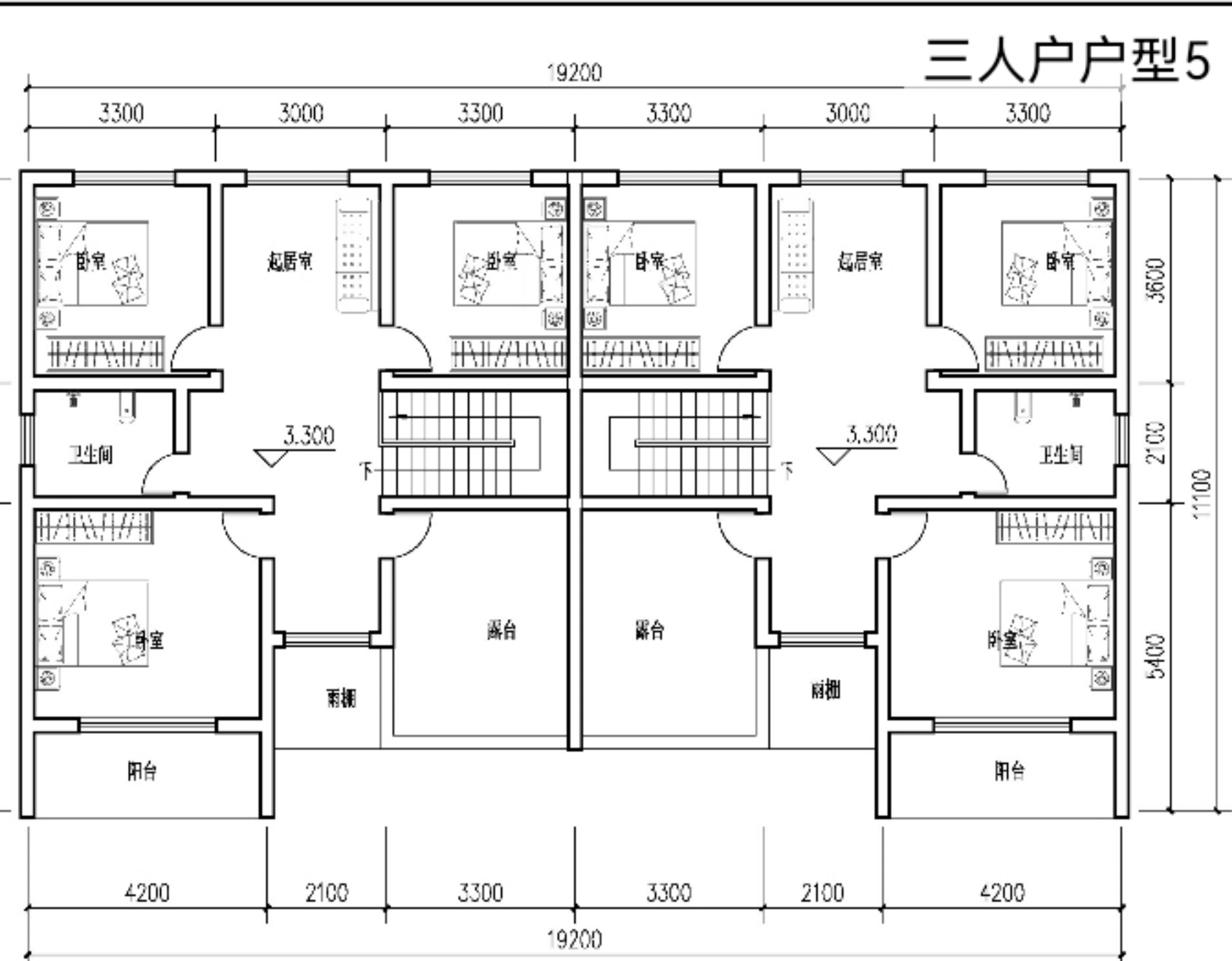
二层平面图 1:100
