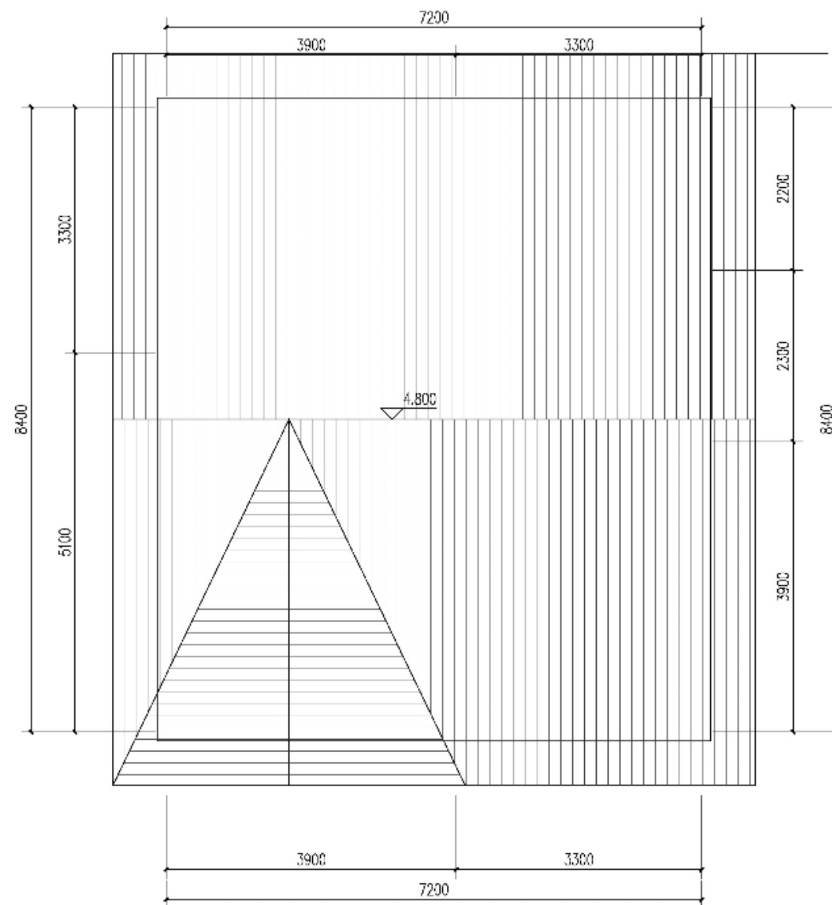
屋顶层平面图 1:50
