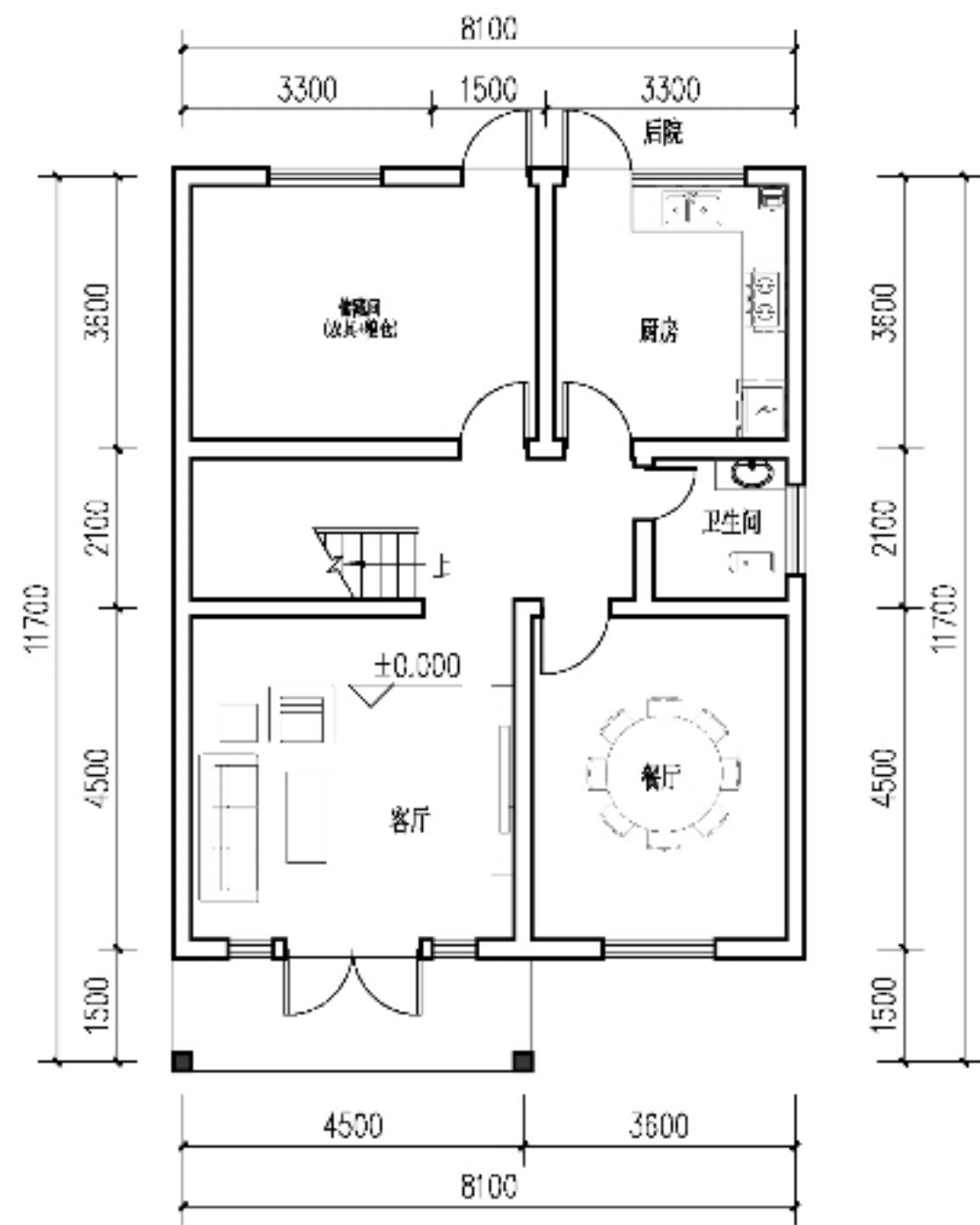
一层平面图 1:100 本层建筑面积: 94.18m 2
