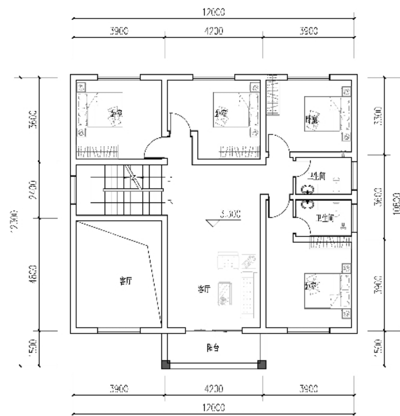
二層平面圖 1:100
