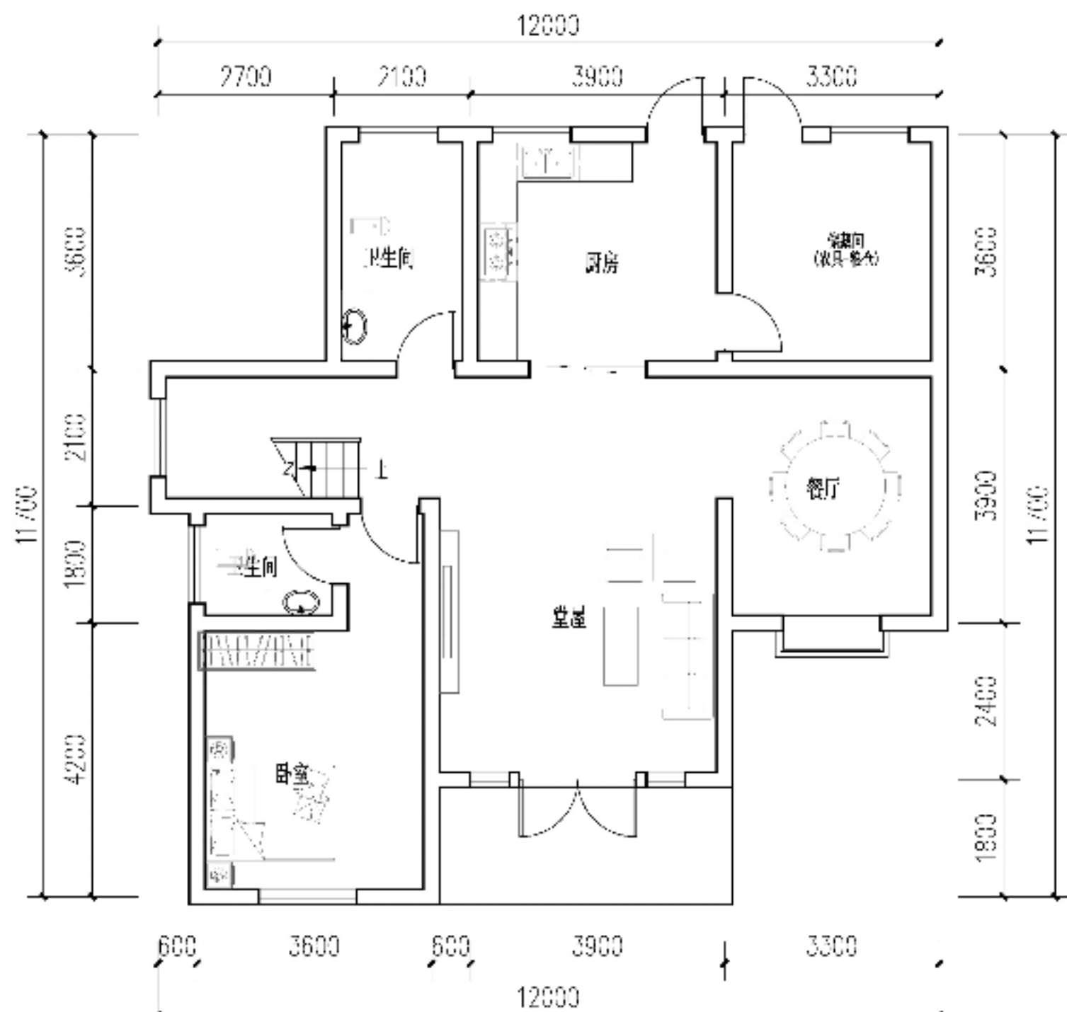
一层平面图 1:100
