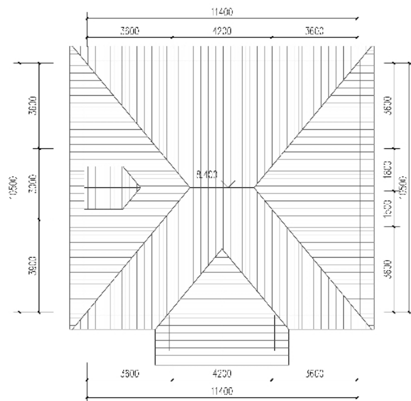
屋顶层平面图 1:100
