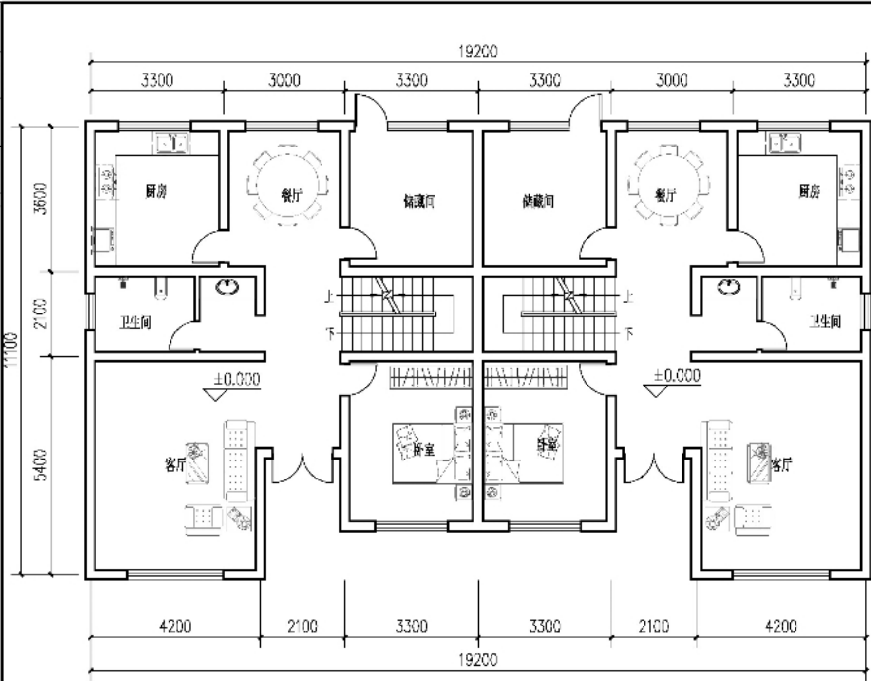
一层平面图 1:100
