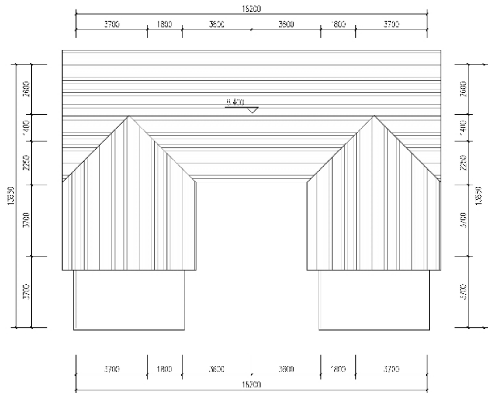
二层平面图 1:100
