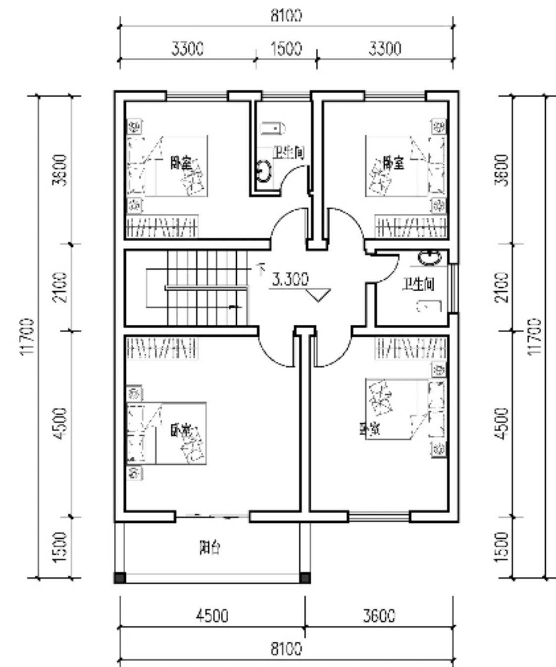
二层平面图 1:100 本层建筑面积: 94.18m 2
