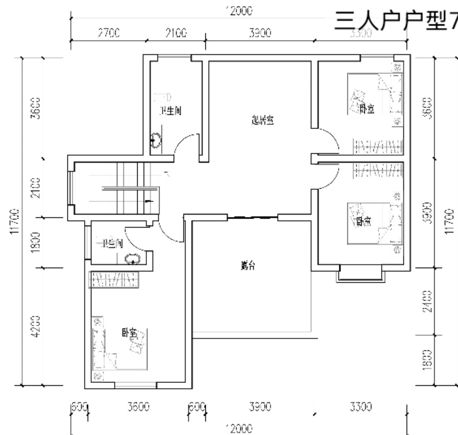
二层平面图 1:100
