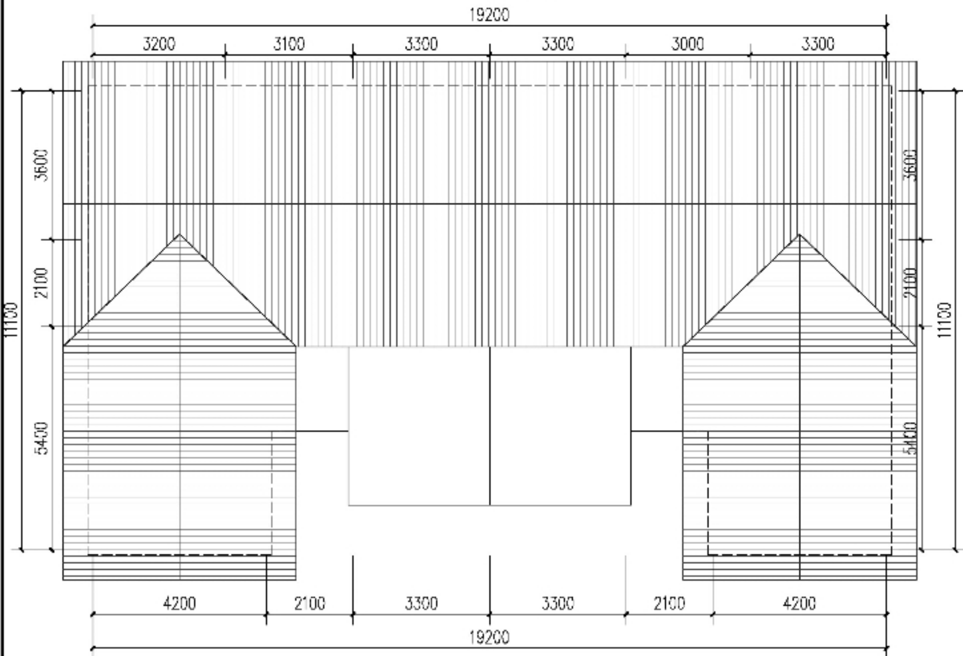
屋顶层平面图 1:100
