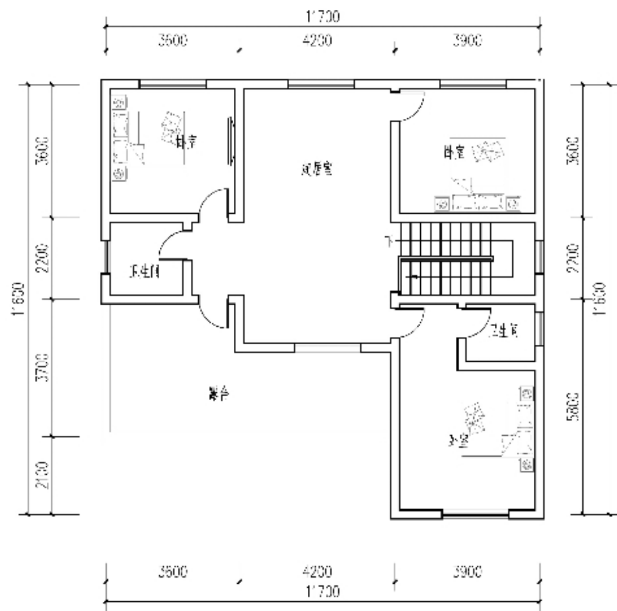
二层平面图 1:100 本层建筑面积: 101.59m 2
