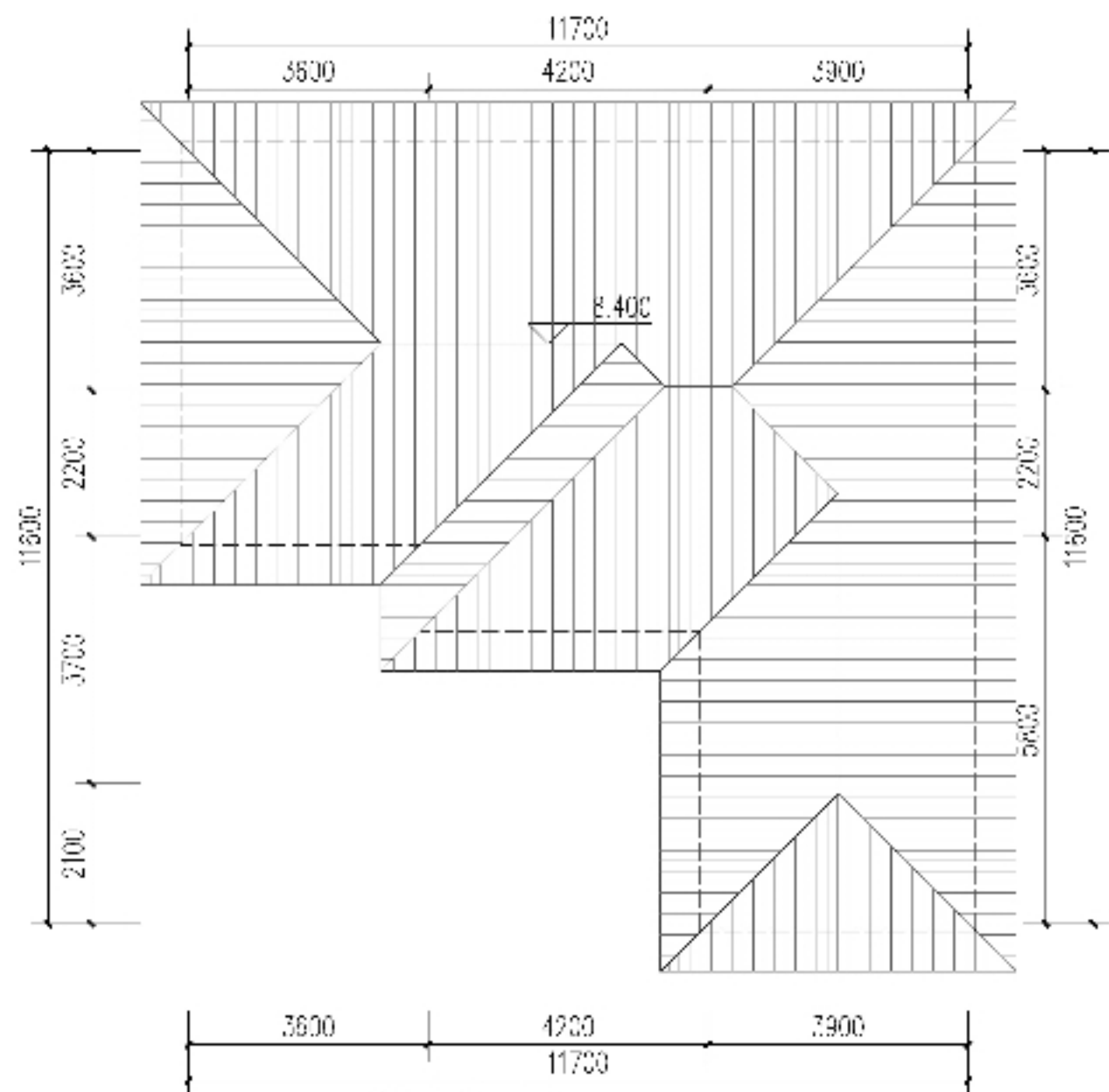
屋顶层平面图 1:100
